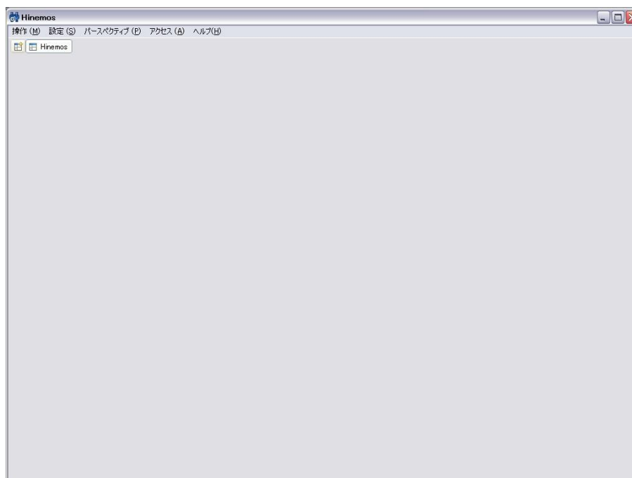
図 6-8 初期画面
