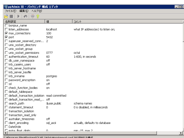
図 36 PostgreSQL の設定ダイアログ
